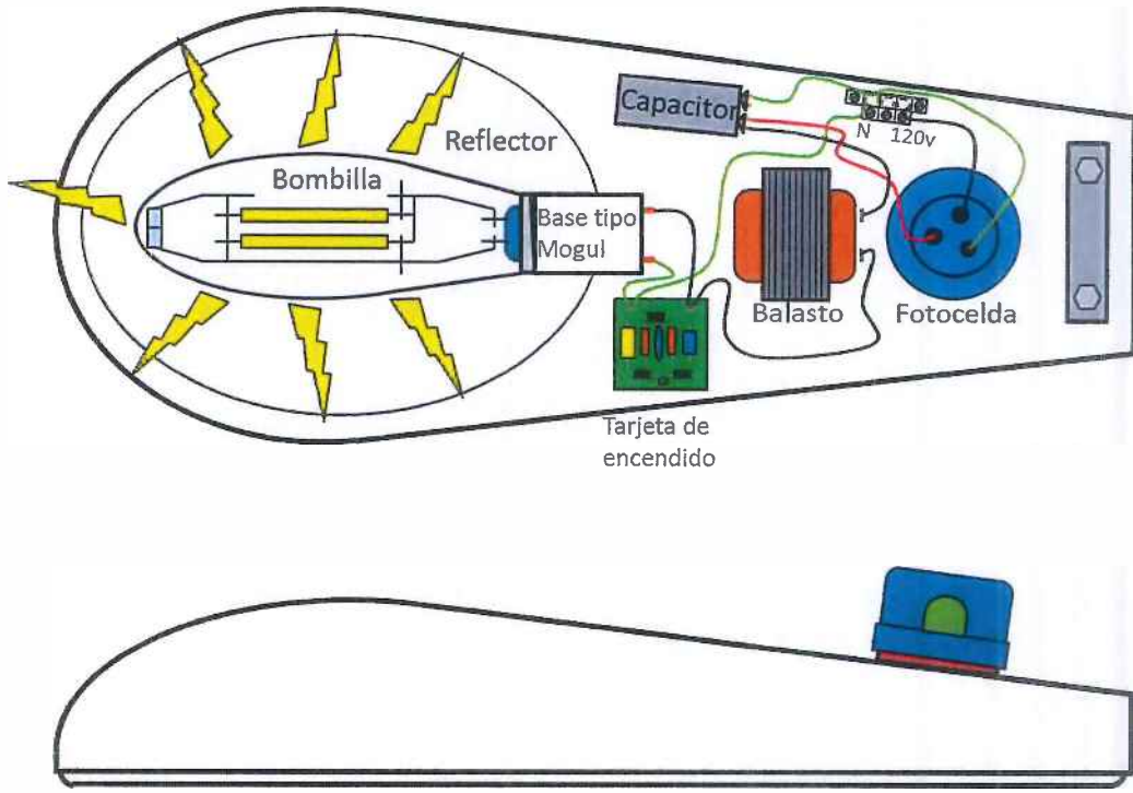
Diagrama de Luminaria con sus Componentes
